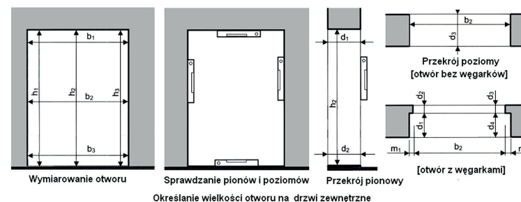
Rys. 2 Wymiarowanie ościeża w ścianie: bez węgarka, z węgarkiem.
