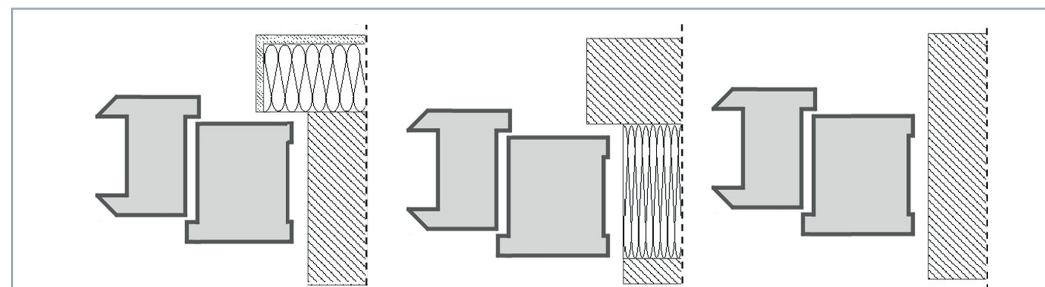
Rys. 3 Usytuowanie ościeżnic w ościeżu ścian różnej konstrukcji: w ścianie pełnej jednowarstwowej, w ścianie warstwowej z ociepleniem wewnętrznym [z węgarkiem], w ścianie pełnej z ociepleniem zewnętrznym [z węgarkiem].
