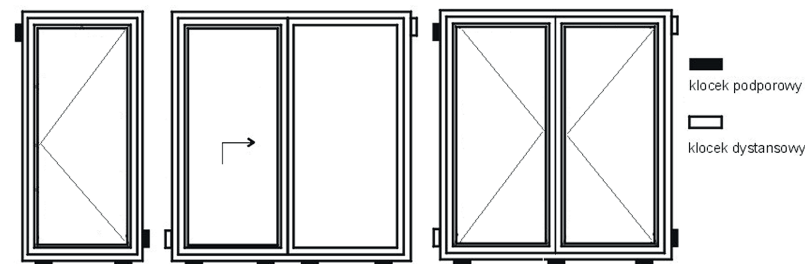
Rys. 1 Usytuowanie klocków / klinów dystansowych do ustalenia pozycji stolarki.
