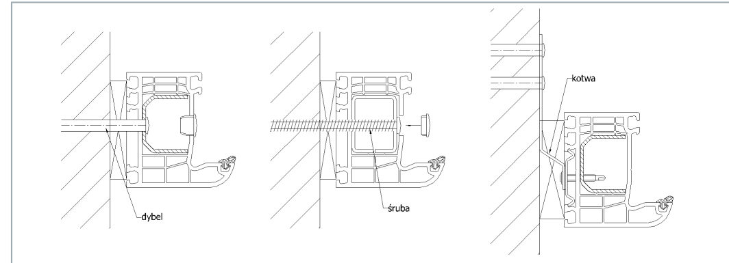
Rys. 5 Rodzaje łączników mechanicznych.
