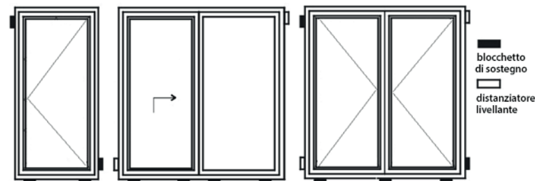
Disegno 1 Posizionamento di blocchetti / distanziatori in funzione della posizione del serramento.
