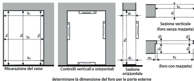
Disegno 2 Misurazione del foro: senza mazzetta, con mazzetta.
