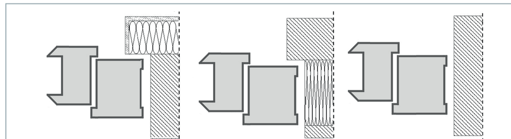
Disegno 3 Posizione dei fori in diversi tipi di strutture: in un muro singolo, in un muro a più strati con isolamento interno [con mazzetta], in un muro pieno con isolamento esterno [con mazzetta].
