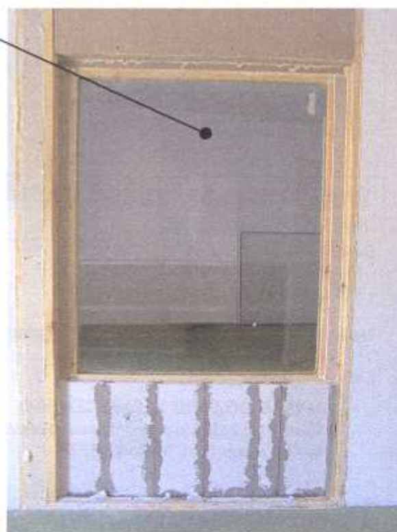
Zdjęcie nr 2 Pakiet szklany typu 6 x 16WES (Argon) x 6 na stanowisku badawczym (widok od strony komory odbiorczej)
